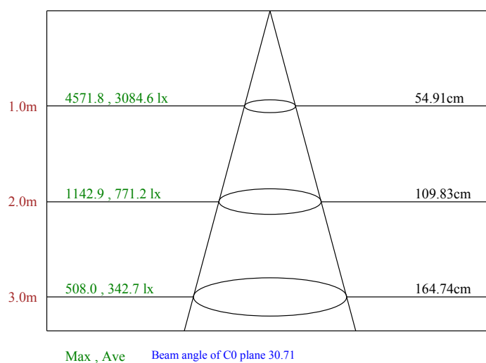
Diagramma conico
